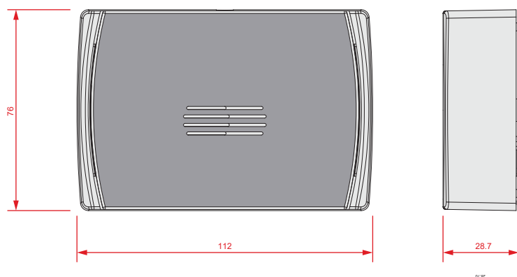
Sounderflasher - dimensions
