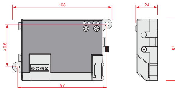
Nexus, Nexus/G, Nexus/3GU - dimensions
