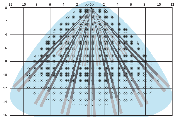
QDT200H, QDT200HM – Top view
