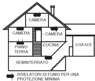
Figura 2: Posizionamento dei rivelatori di fumo e di calore in una abitazione su più livelli
