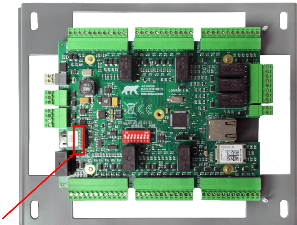
Connecteur du Dongle
