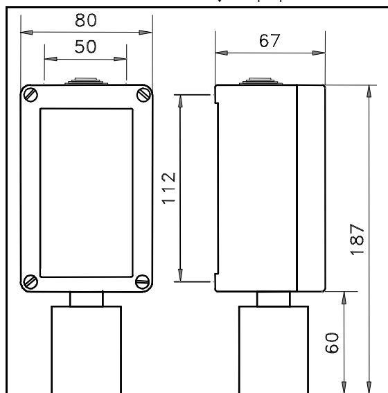
Fig. 1 - Dimensioni / Size / Dimensions
