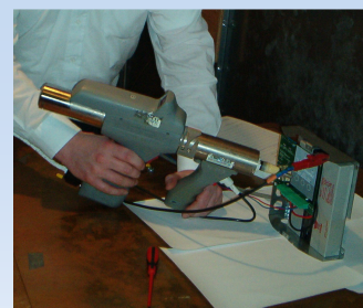
ESD gun test
